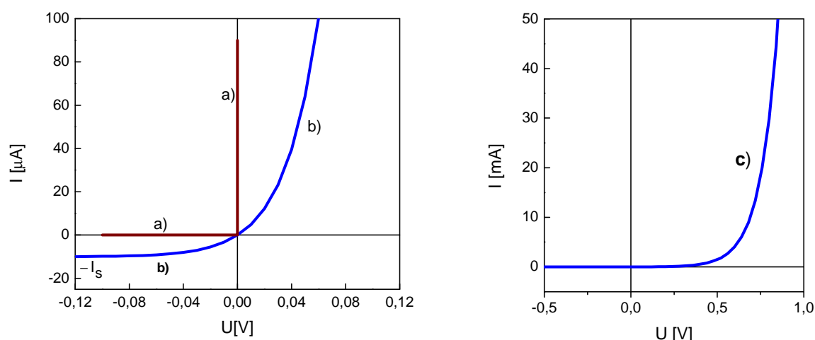
Rys. 3. Charakterystyki teoretyczne: a) „dioda idealna” (sprzeczna z zasadami fizyki), b) ch-ka obliczona z wzoru Shockleya, przyjmując I_s = 10 \mu\text{A} i T = 300 \text{ K} , c) ta sama charakterystyka pokazana w większym przedziale prądów i napięć
